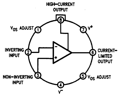
TL/H/9414-2
