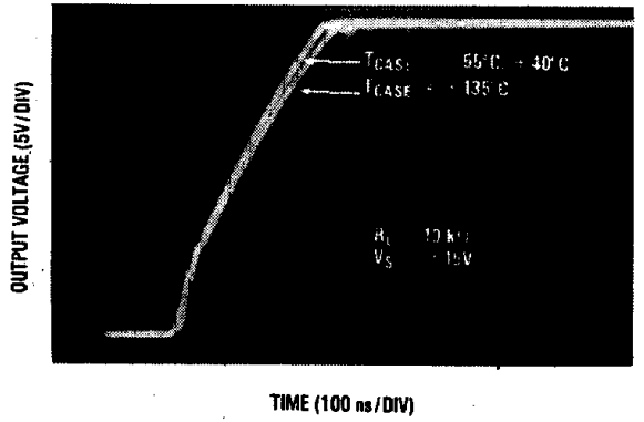
TL/H/9414-15
